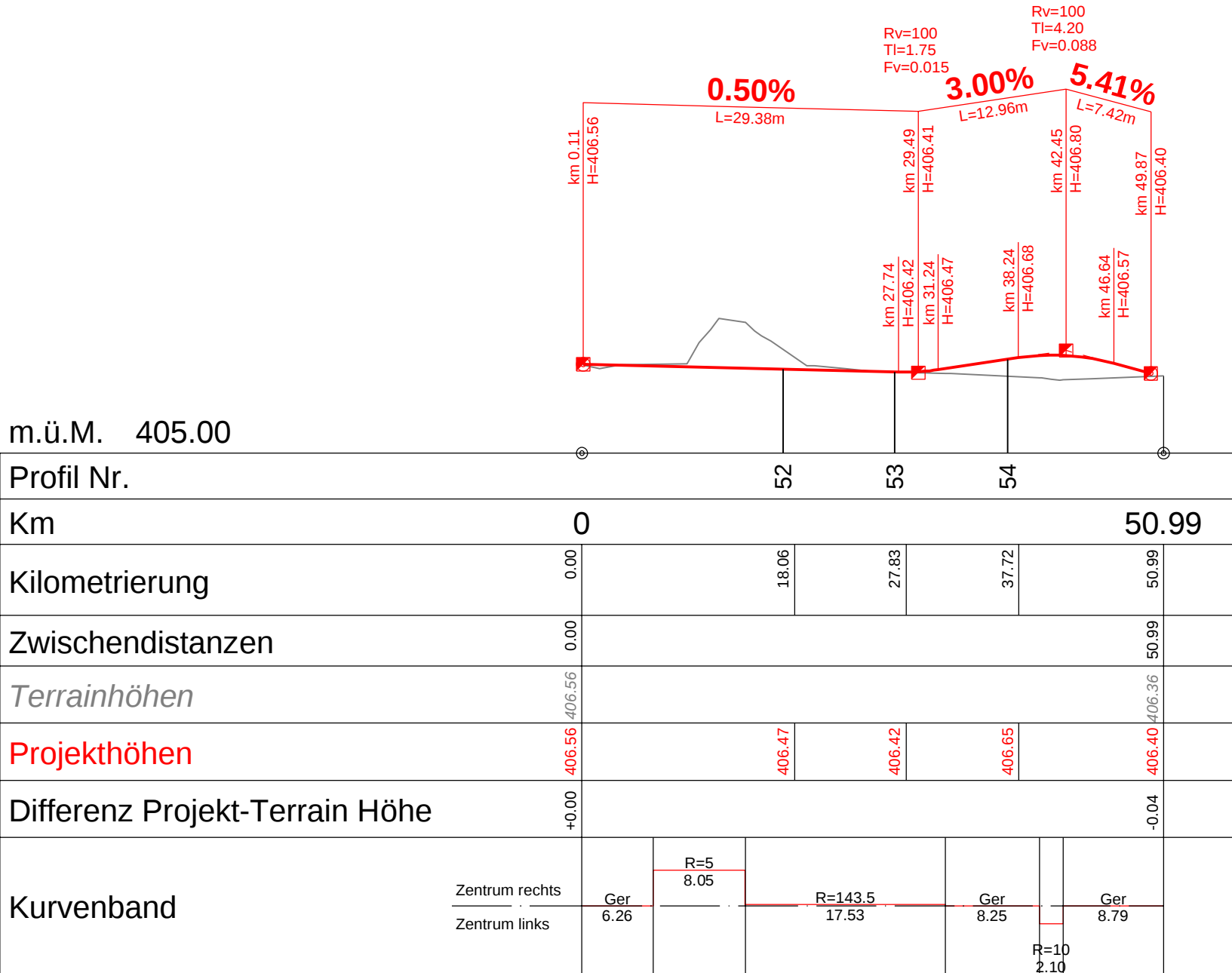
Längenprofil Bachfeldweg:
